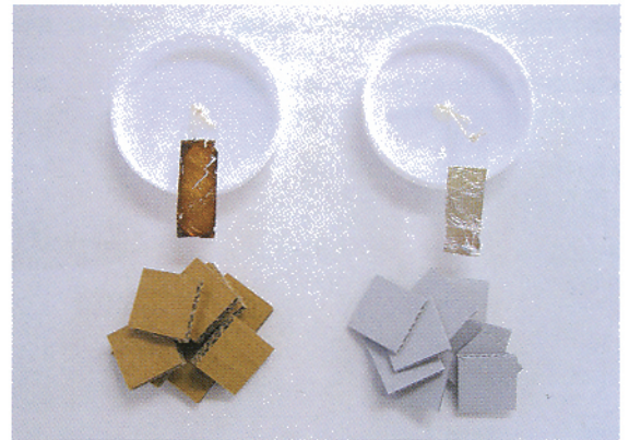
▲比較実験結果。密閉ガラスびんにそれぞれ普通の段ボール(左)とアーカイバルボード(右)を入れ、銀箔をつるして4か月間放置。左は硫化水素により変色した銀箔、右は変化のない銀箔。
